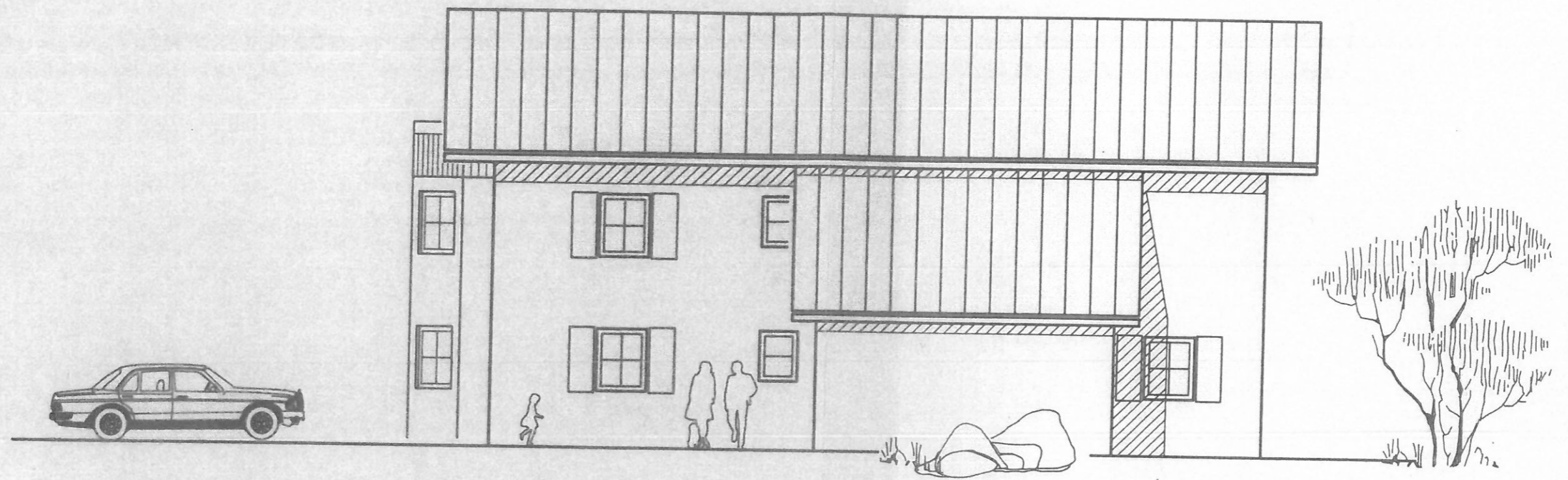
NORDANSICHT
