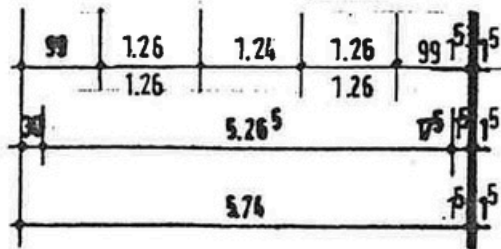
OBERGESCHOSS M. 1: 100
