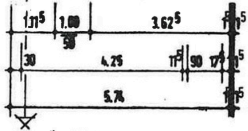
KELLERGESCHOSS M. 1:100
