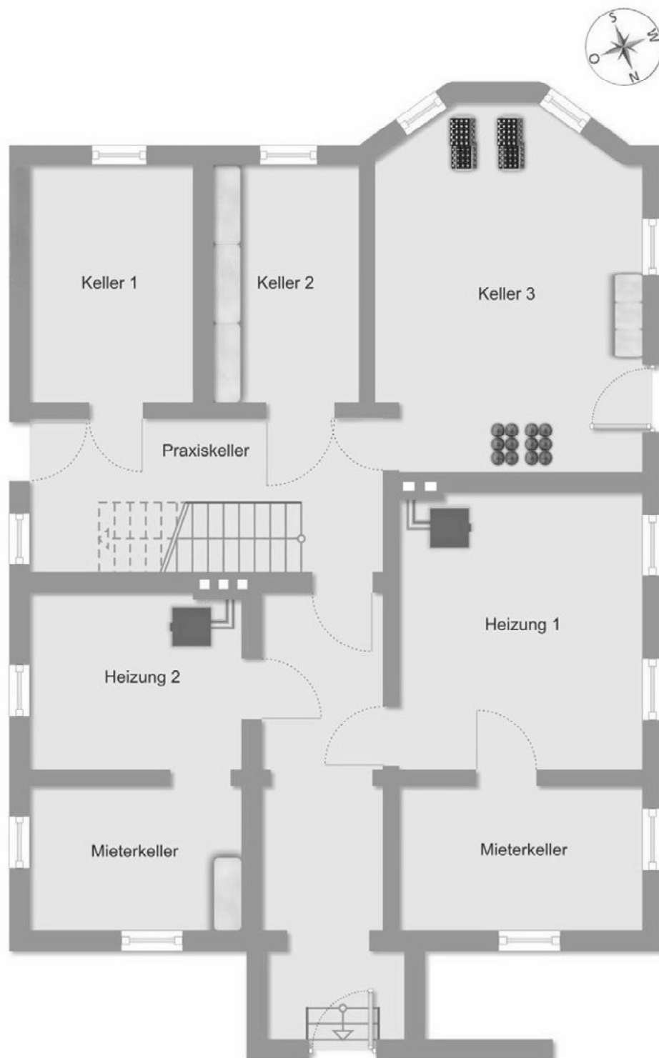
■ Grundriss Keller
