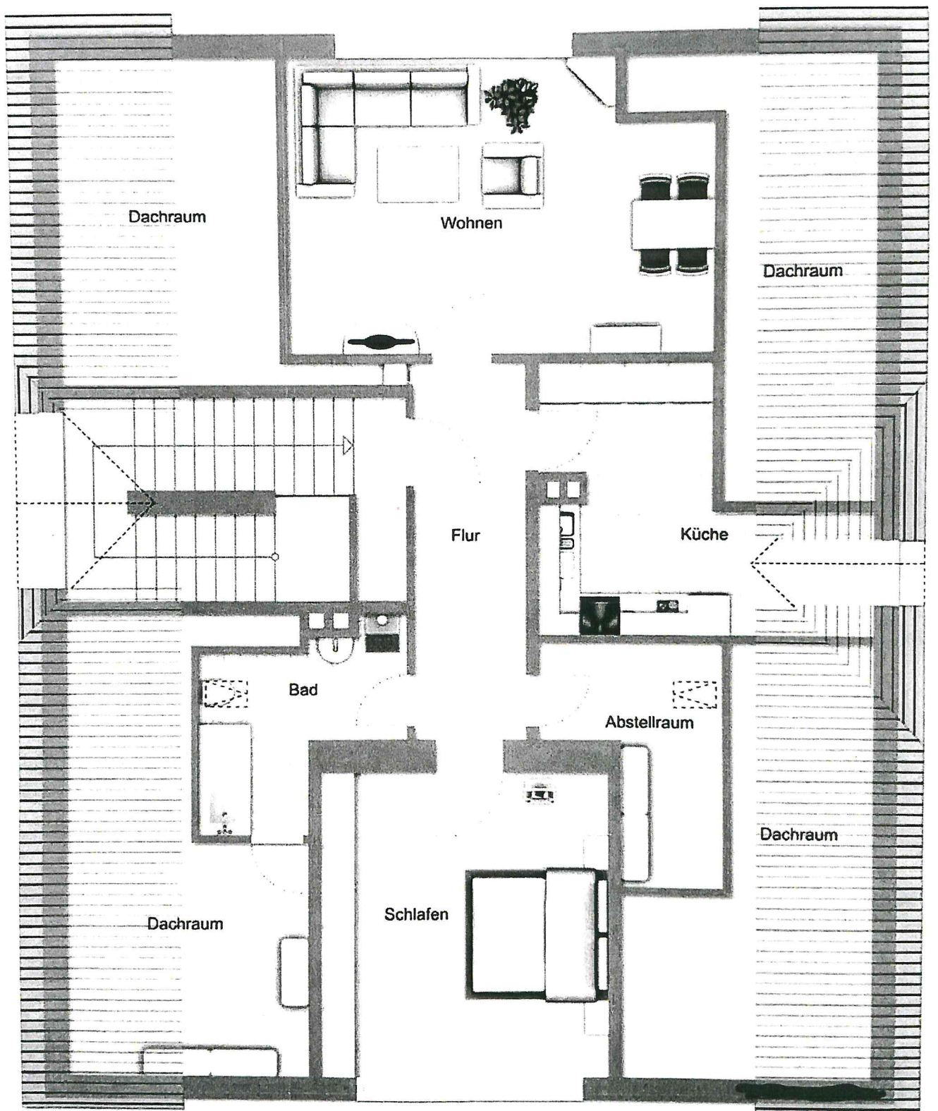
■ Grundriss Dachgeschoss
