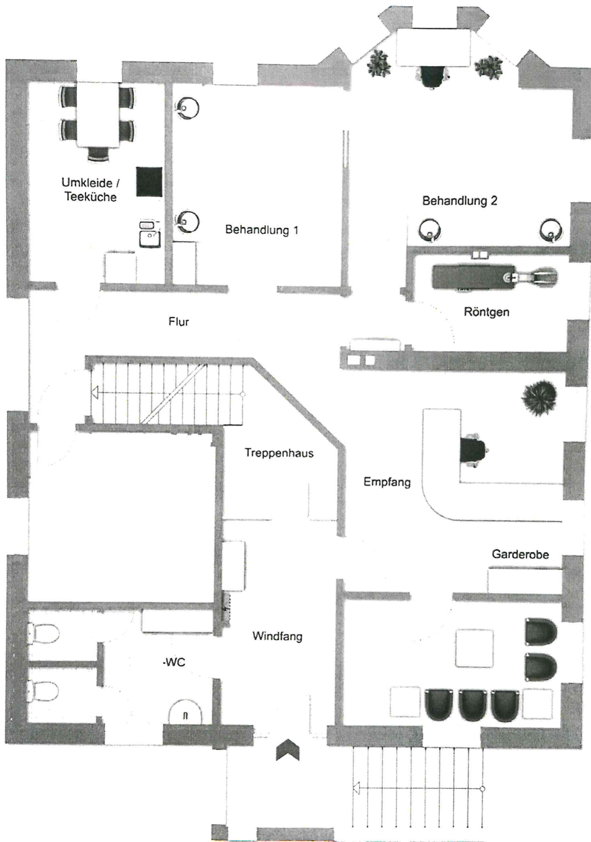
■ Grundriss Erdgeschoss
