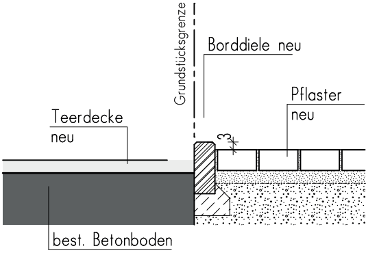
SCHNITT CC
