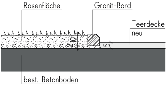
SCHNITT BB
