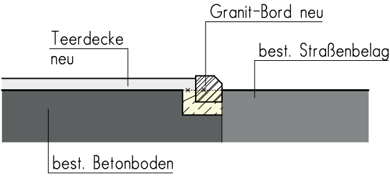
SCHNITT AA
