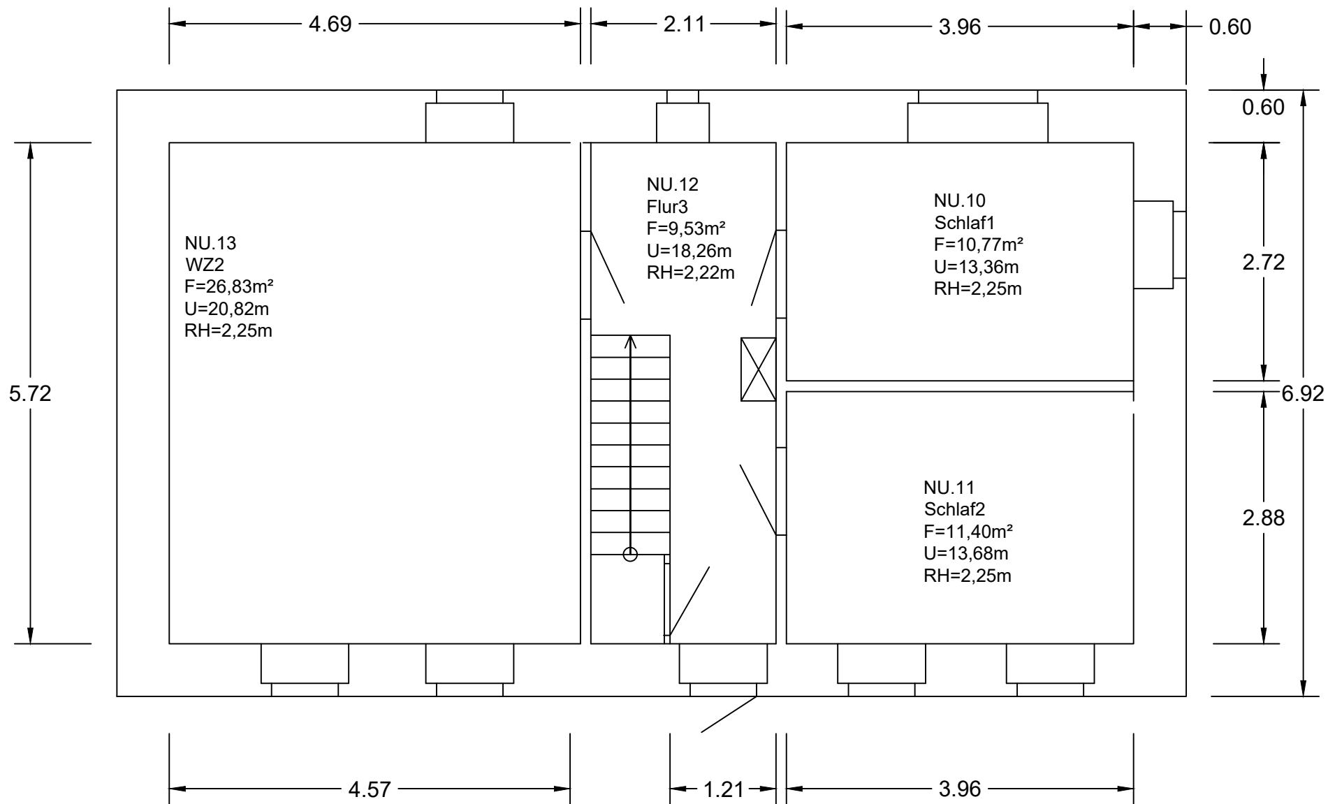
Grundriss OG
