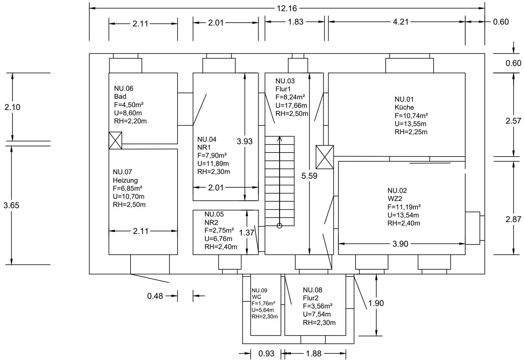
Grundriss EG
