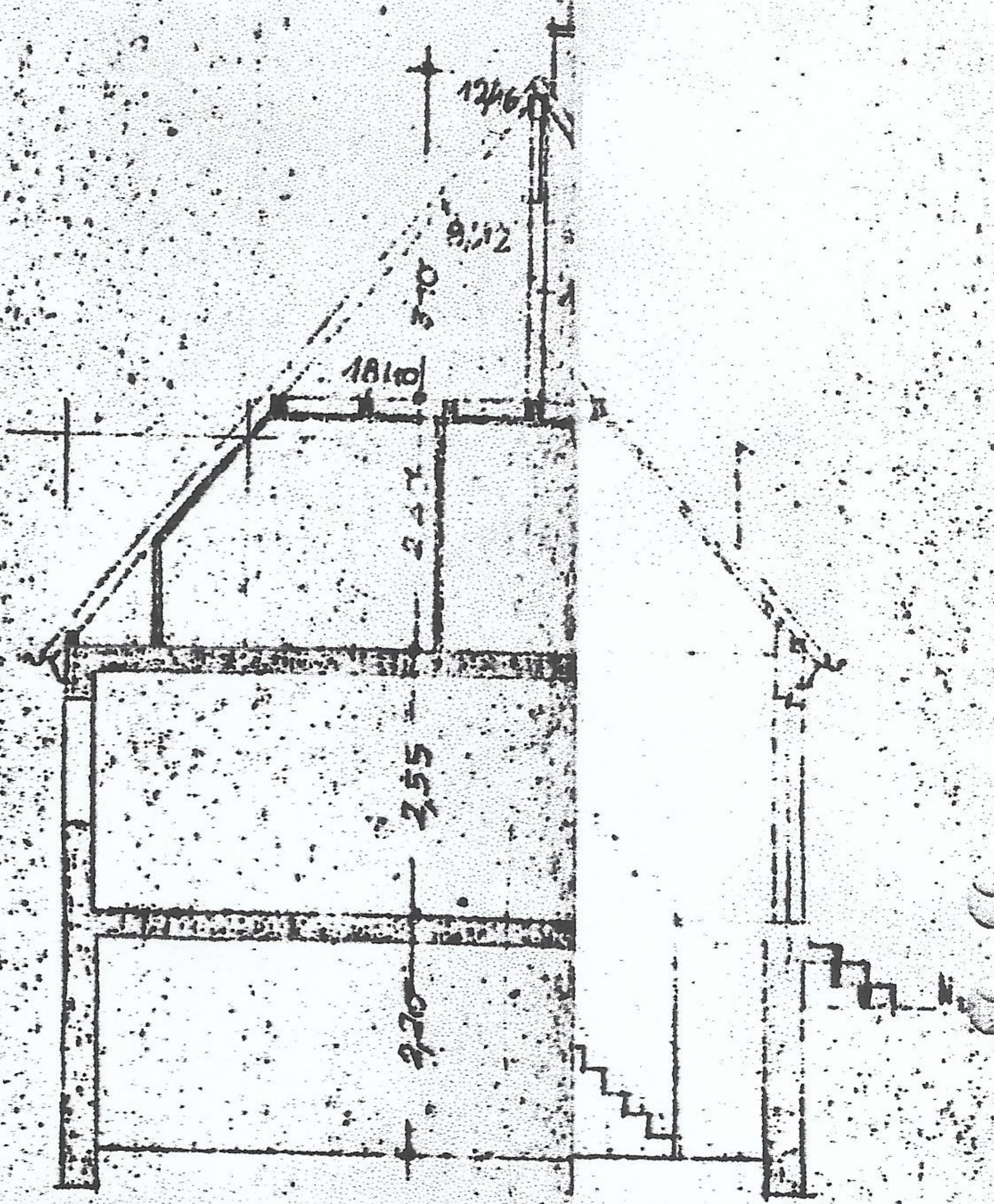
SCHNITT
