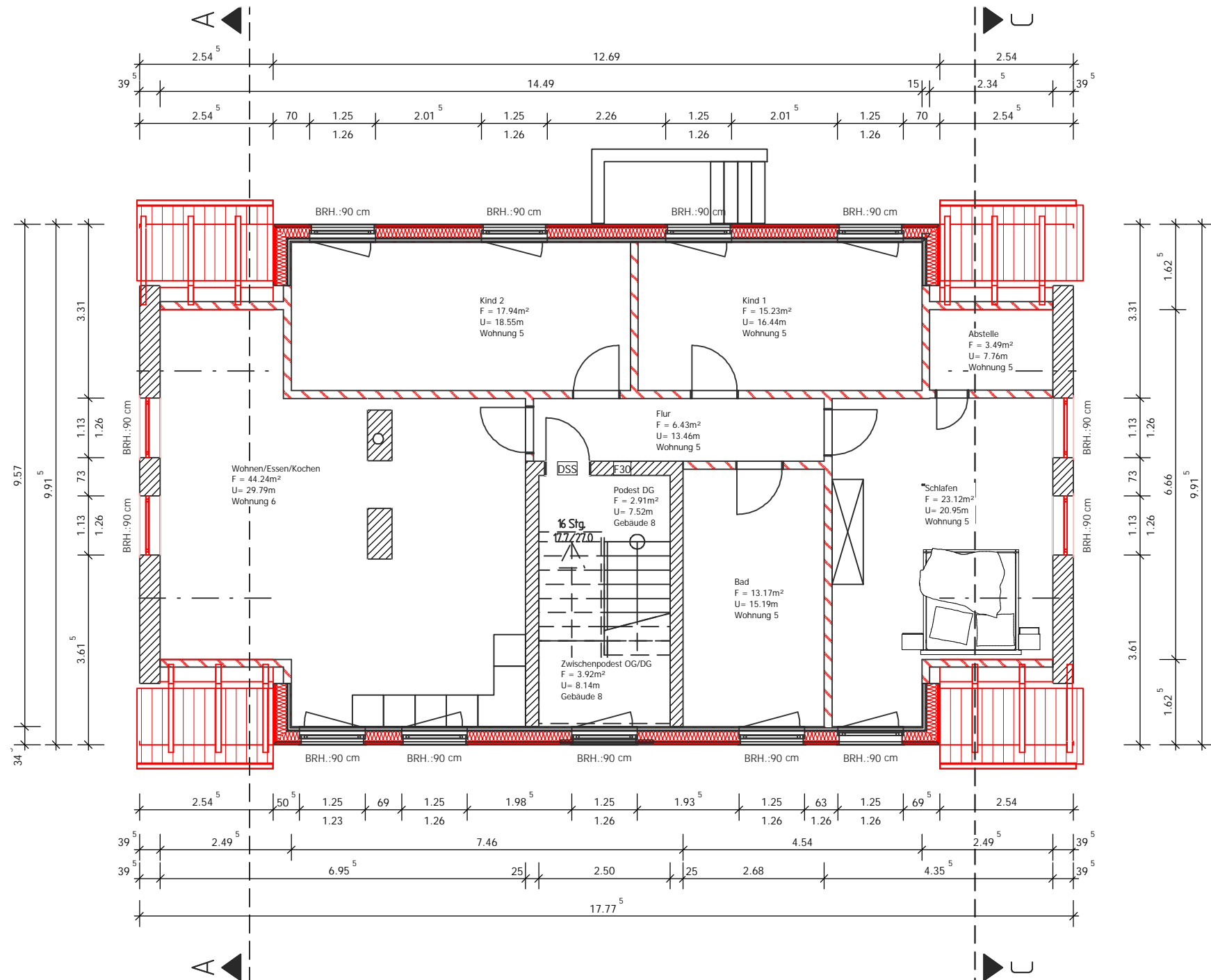
Grundriss Dachgeschoss - Umbau
