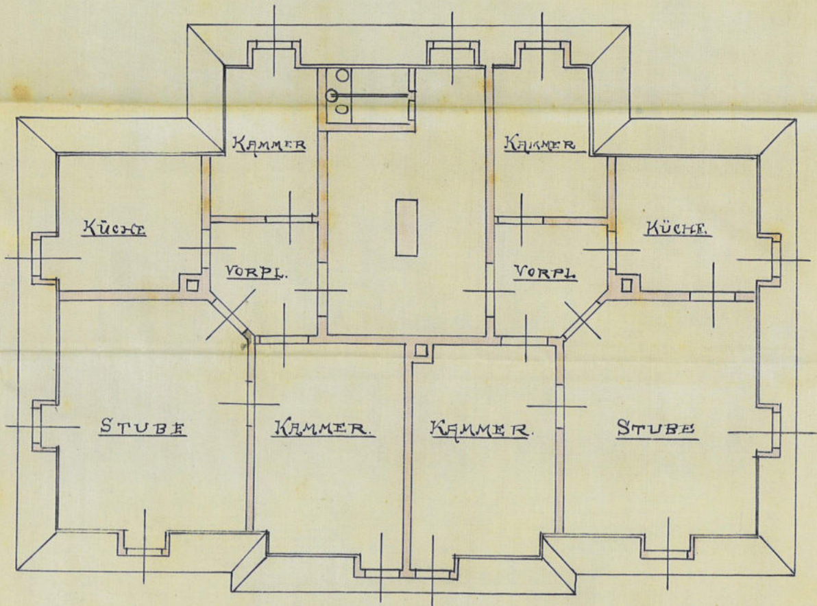
— DACHGESCHOSS —
