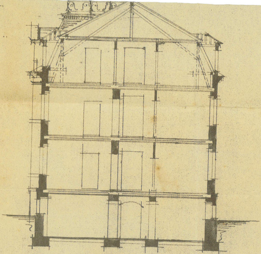
PROFIL
