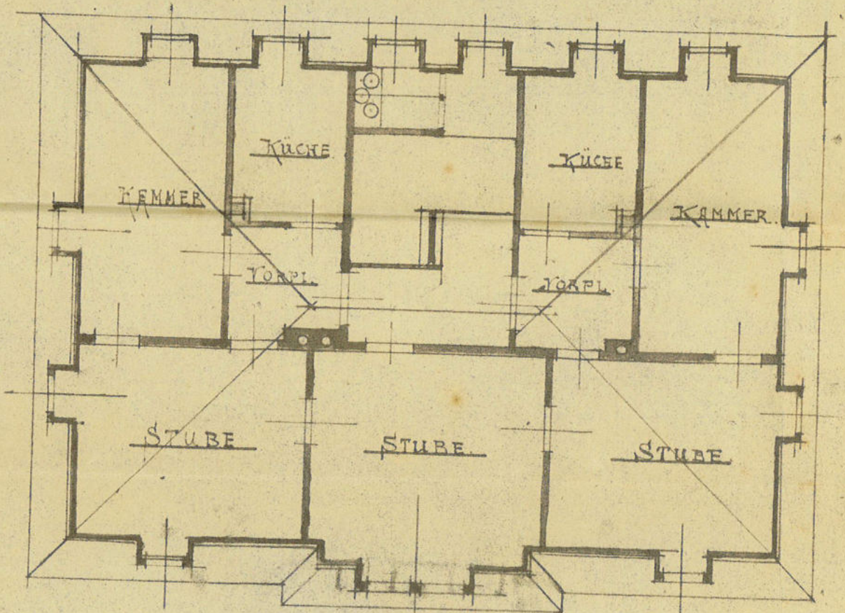
DACHGESCHOSS
