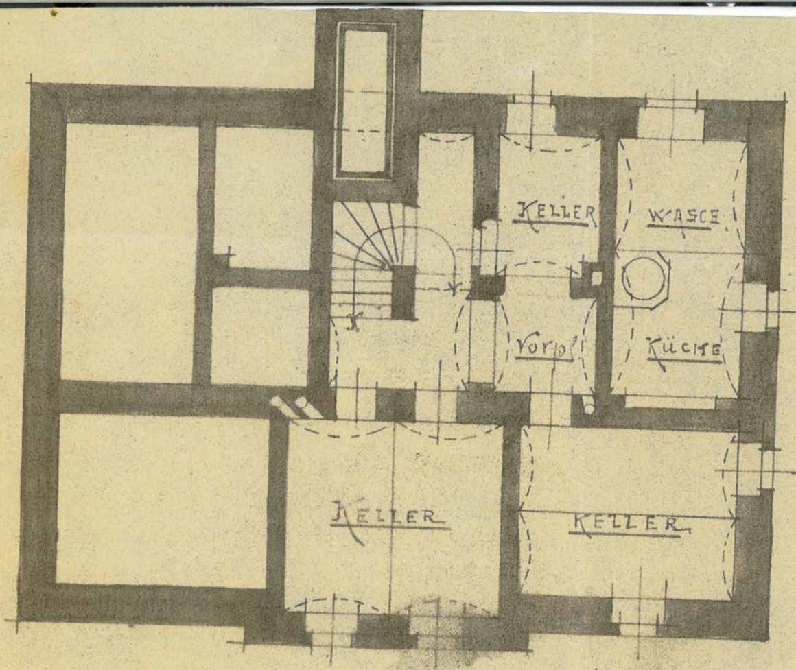
KELLERGEESCHOSS
