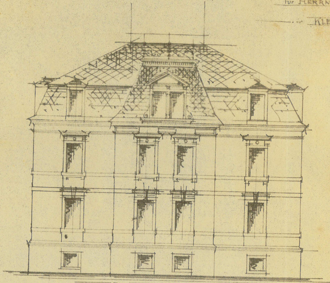
HAUPTANSICHT
