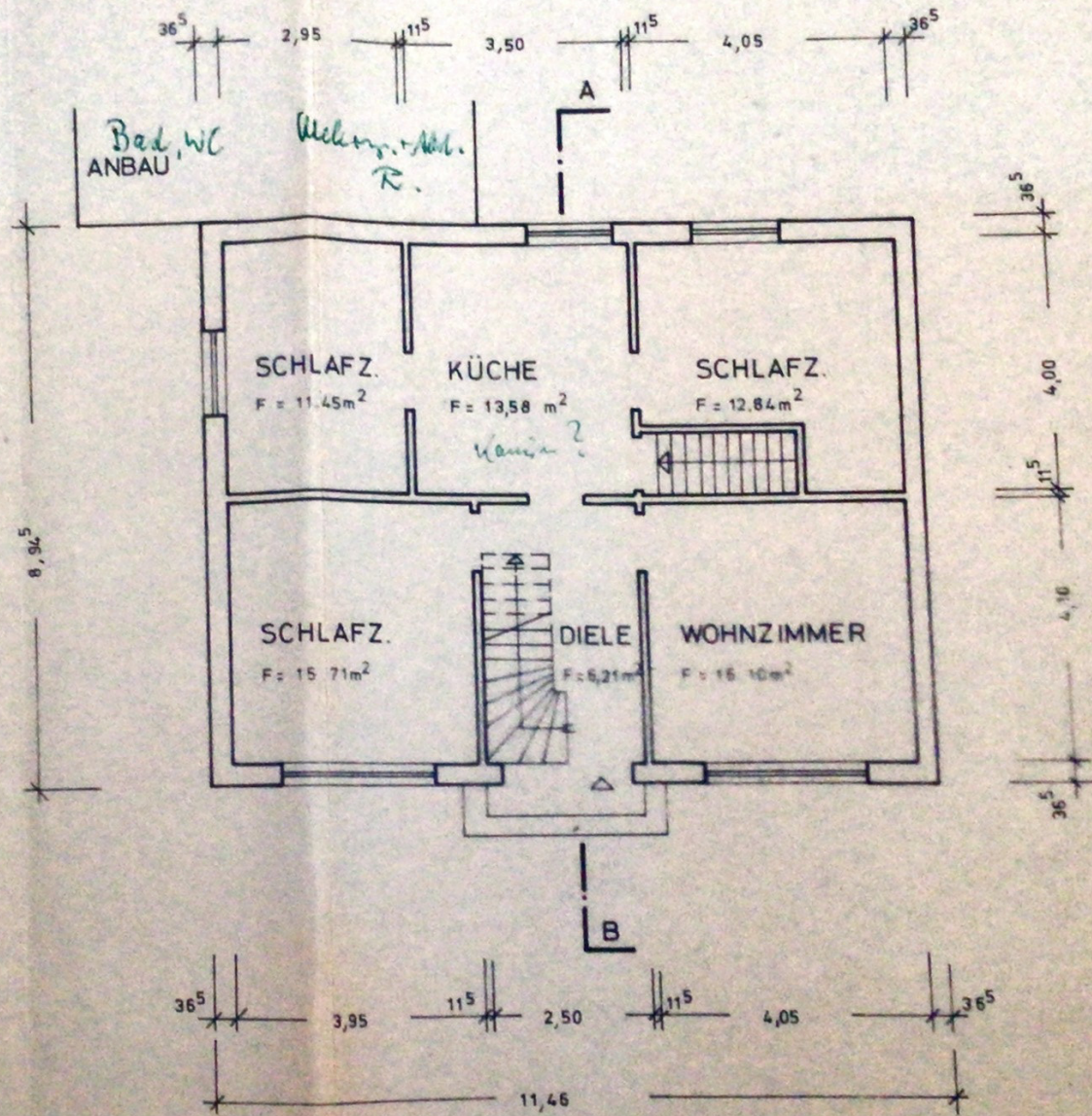
ERDGESCHOSS (VORHANDEN)
