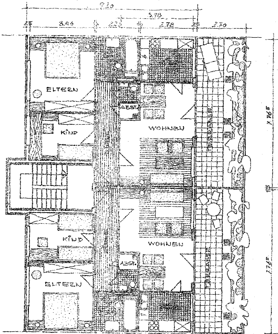
GRUNDRISS ZOBBERGESCHOSS H 1:100 AUSSCHNITT FÜNFERBLOCK
