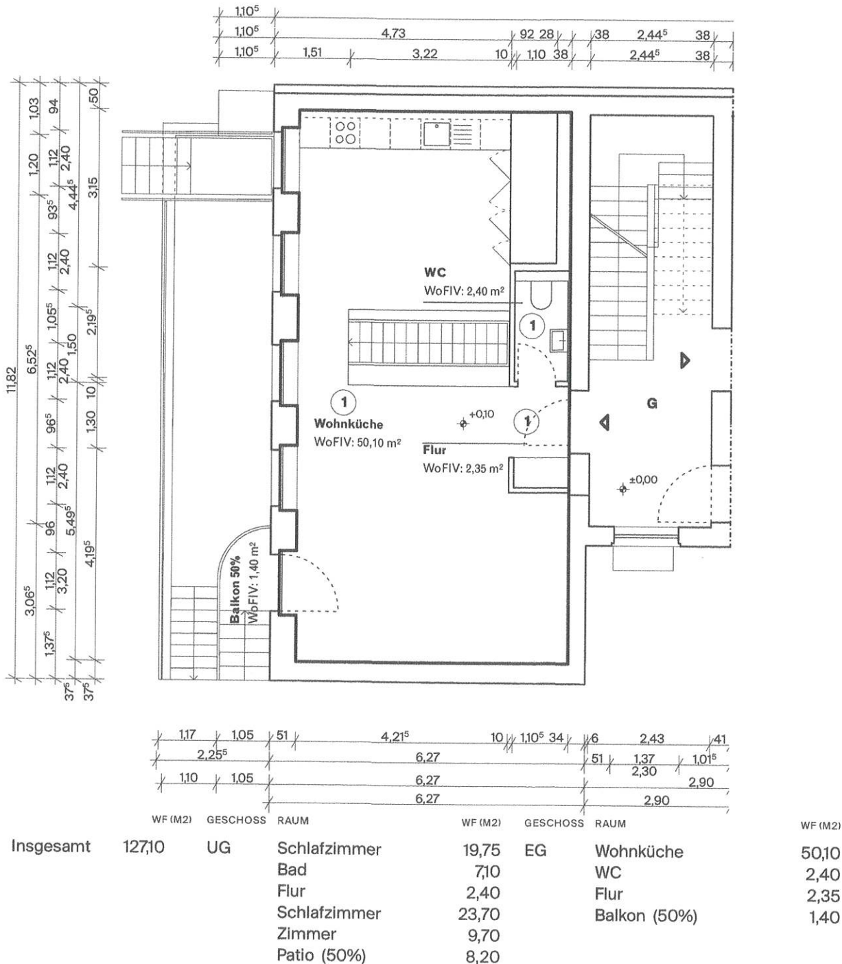
Grundriss Erdgeschoss, M 1:100
