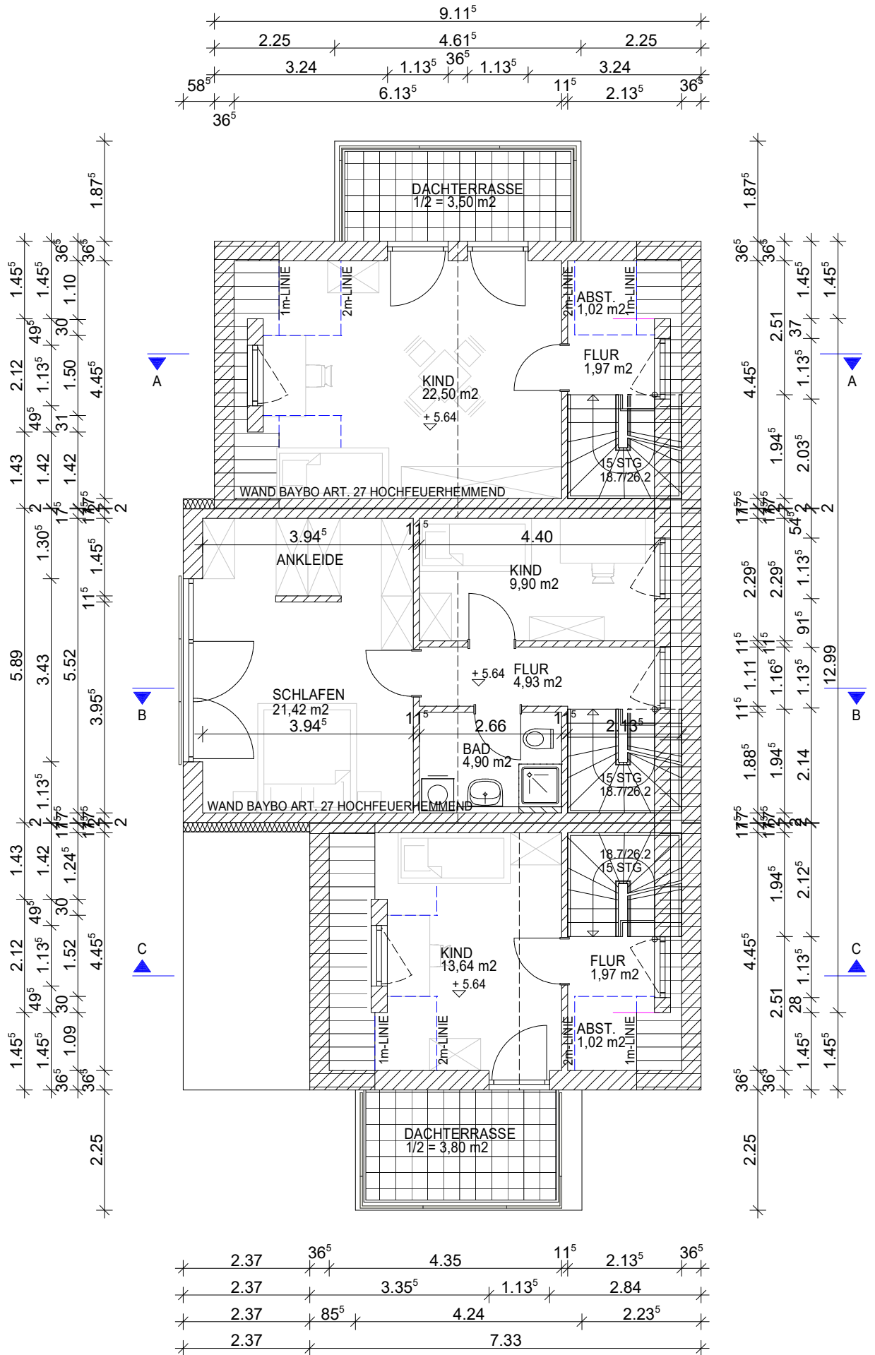
GRUNDRISS DG
