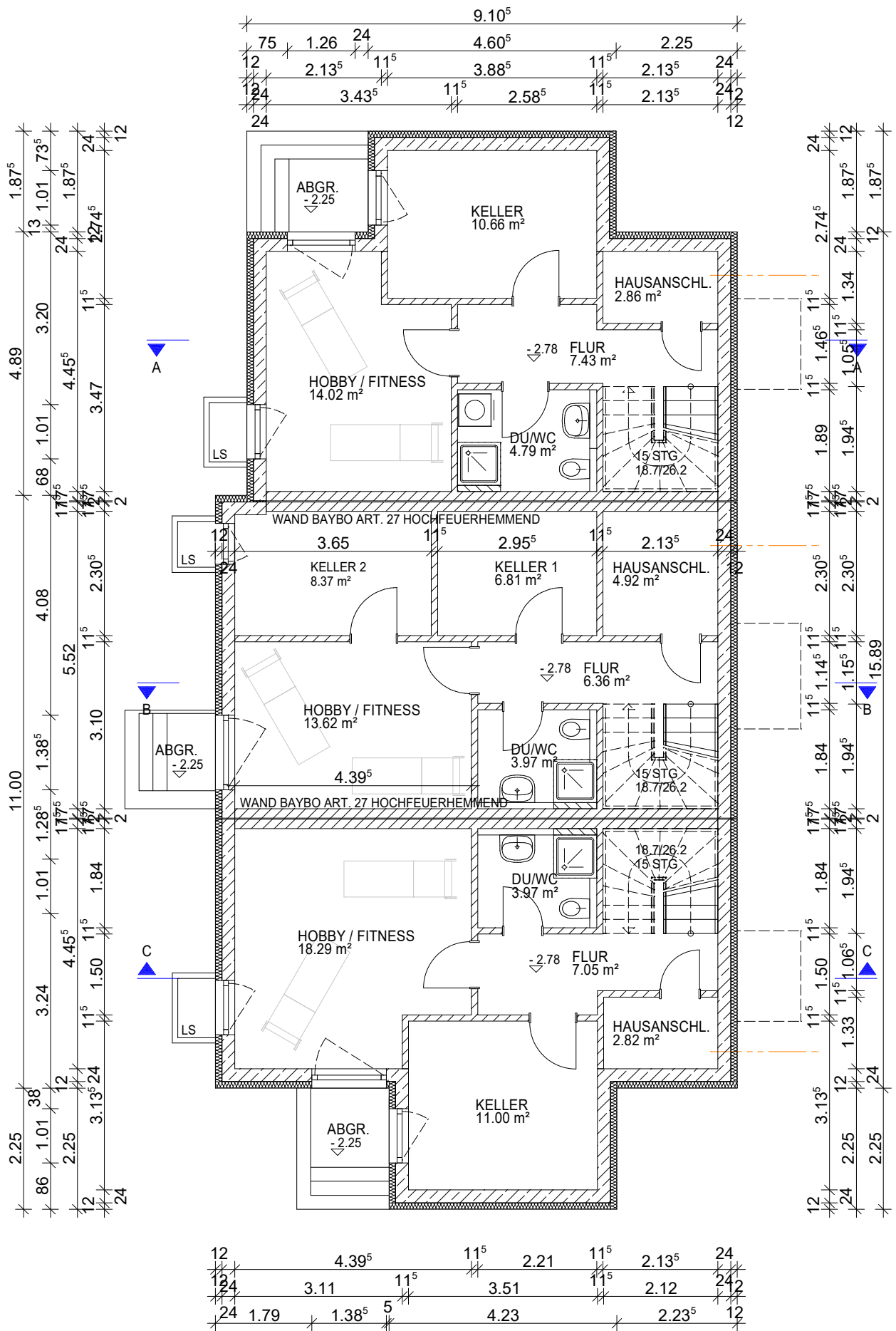
GRUNDRISS UG
