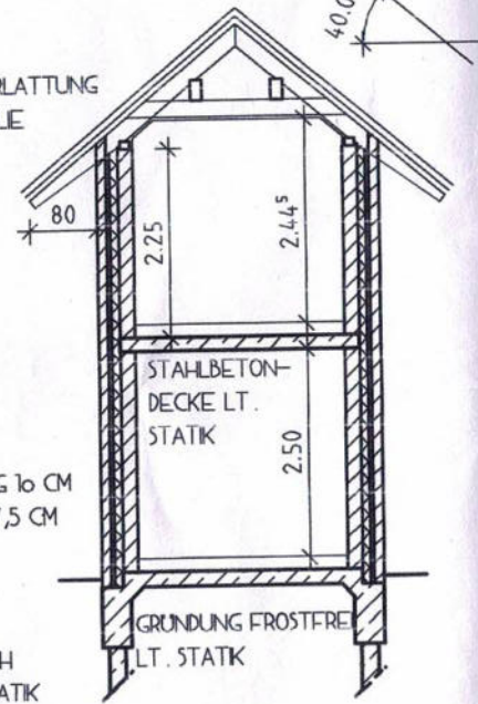
SCHNITT B-B
