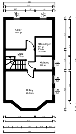
KELLERGESSCHOSS
