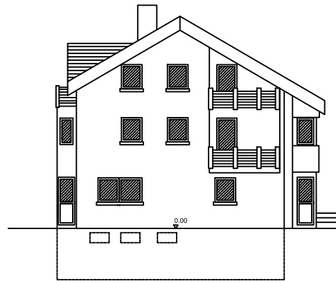
SÜDANSICHT
