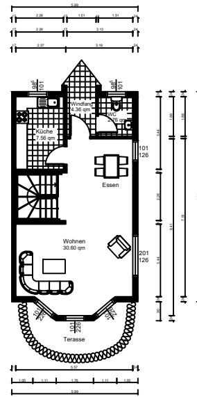
ERDGESSCHOSS
