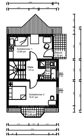
DACHGESCHOSS
