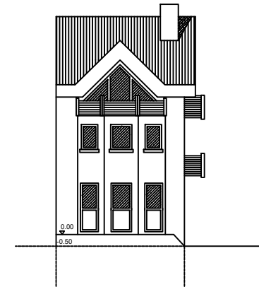
WESTANSICHT
