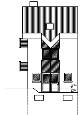
OSTANSICHT
