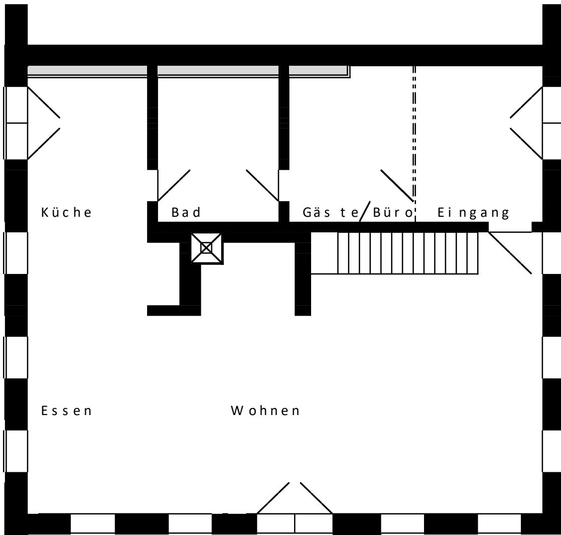
Erdgeschoss Innenmaß ca. 13,50 m x 12 m
