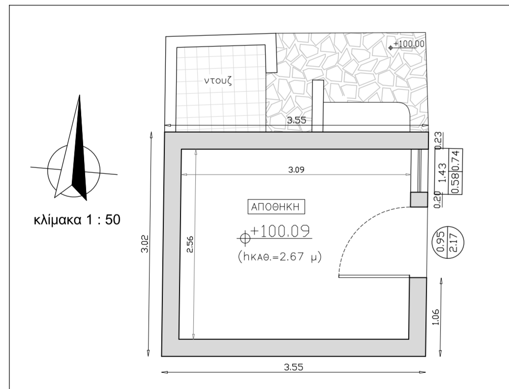
ΚΑΤΟΨΗ ΙΣΟΓΕΙΟΥ ΕΞΩΤΕΡΙΚΗΣ ΑΠΟΘΗΚΗΣ
