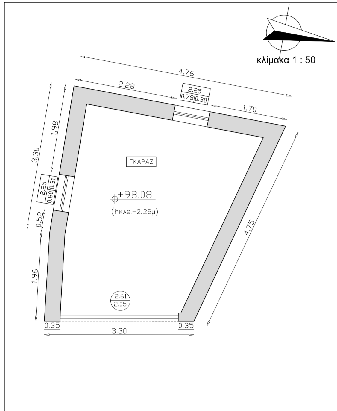
ΚΑΤΟΨΗ ΙΣΟΓΕΙΟΥ ΓΚΑΡΑΖ
