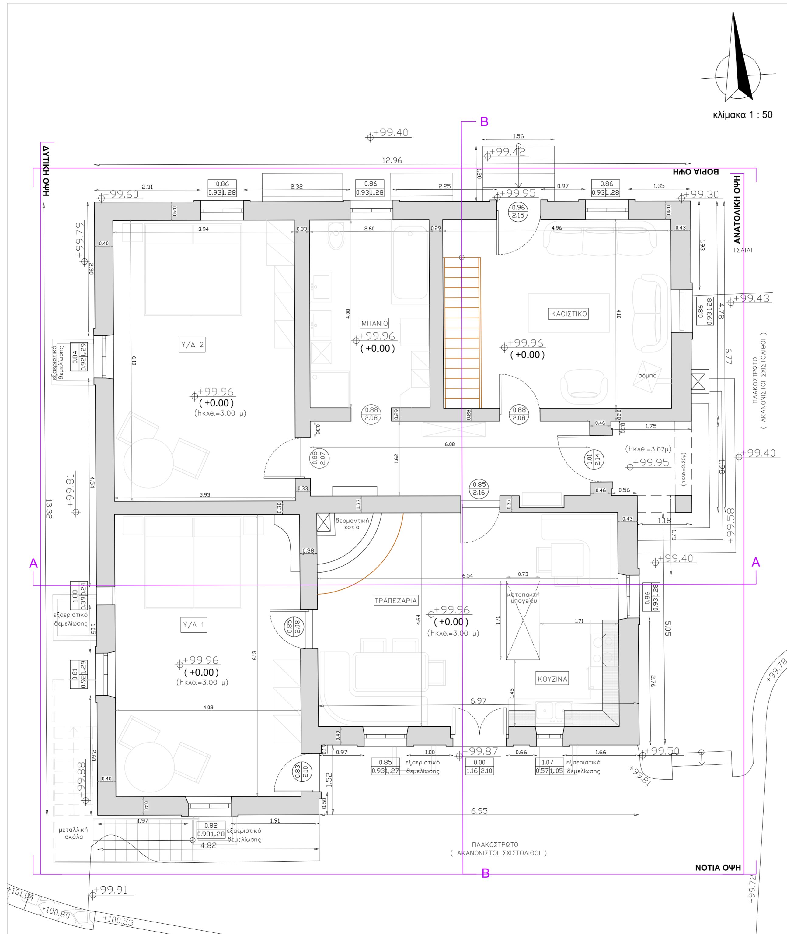
ΚΑΤΟΨΗ ΙΣΟΓΕΙΟΥ ΚΑΤΟΙΚΙΑΣ
