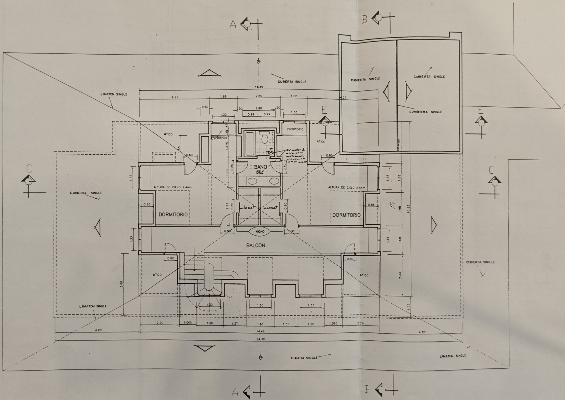
PLANTA DE DISTRIBUCION ARQUITECTONICA PRINCIPAL 2º NIVEL
