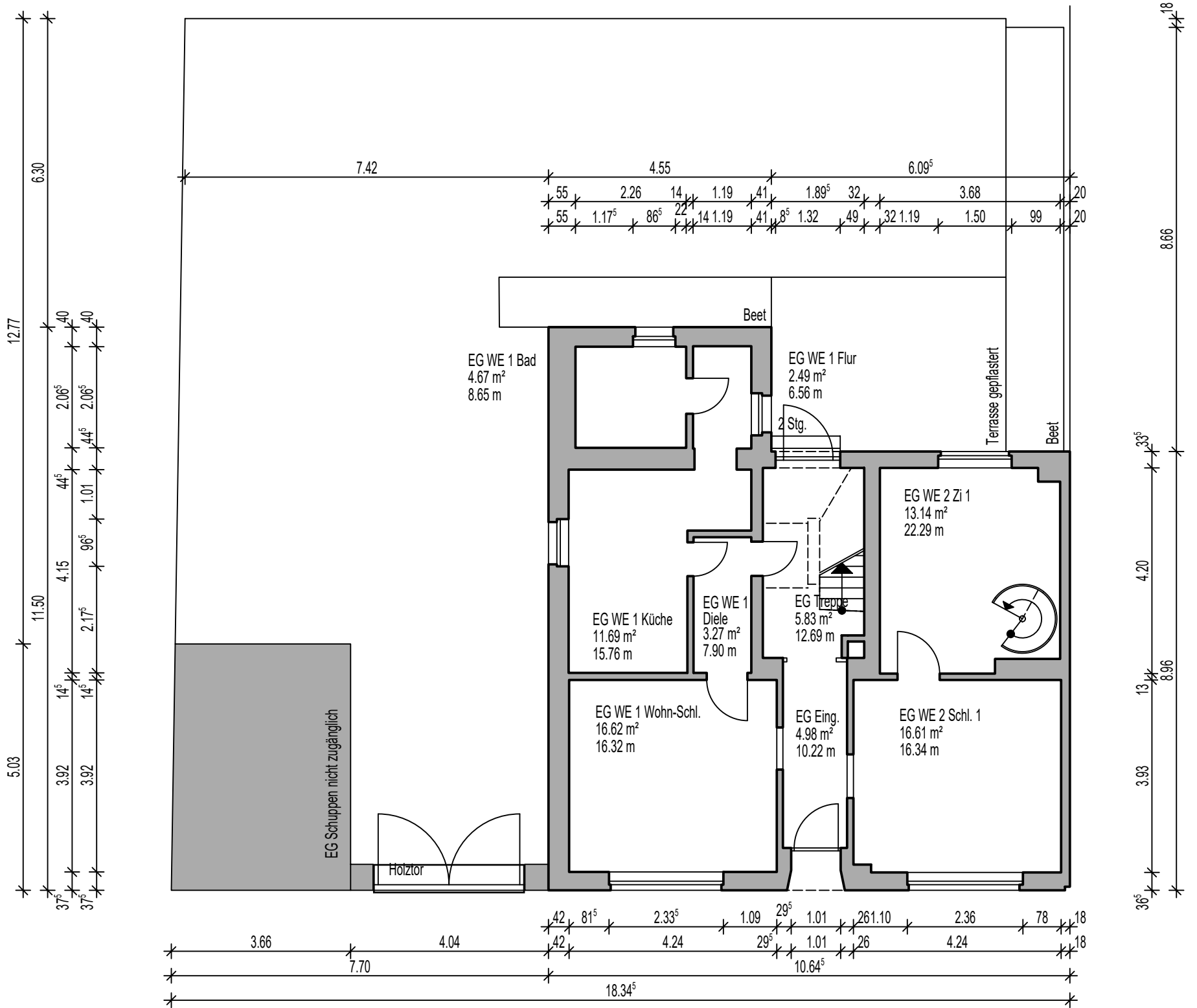
GRUNDRISS EG
