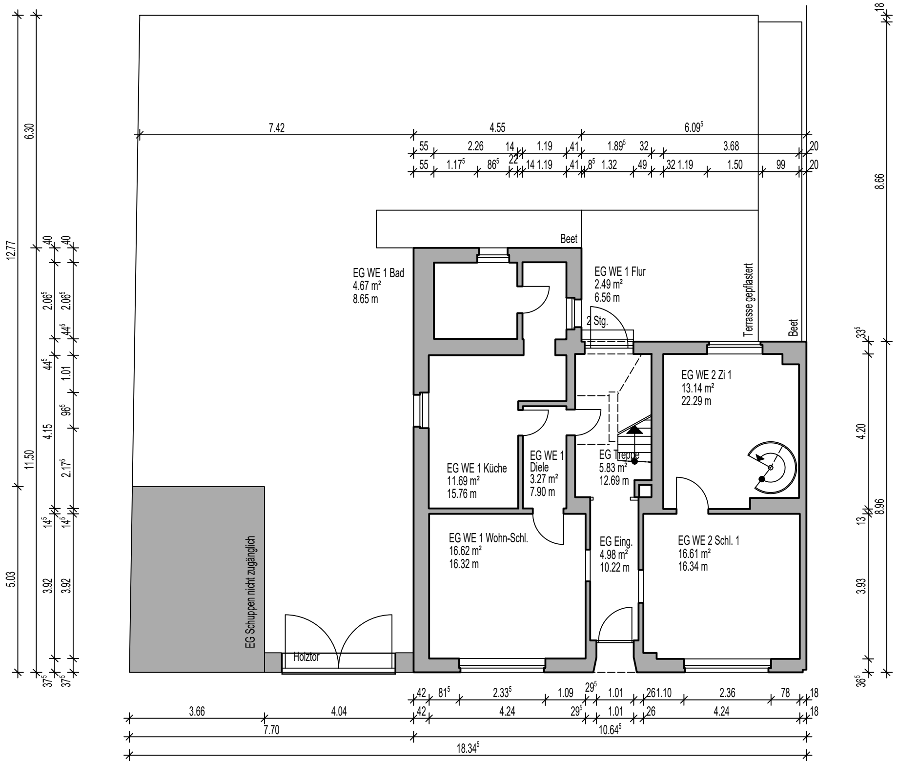
GRUNDRISS EG
