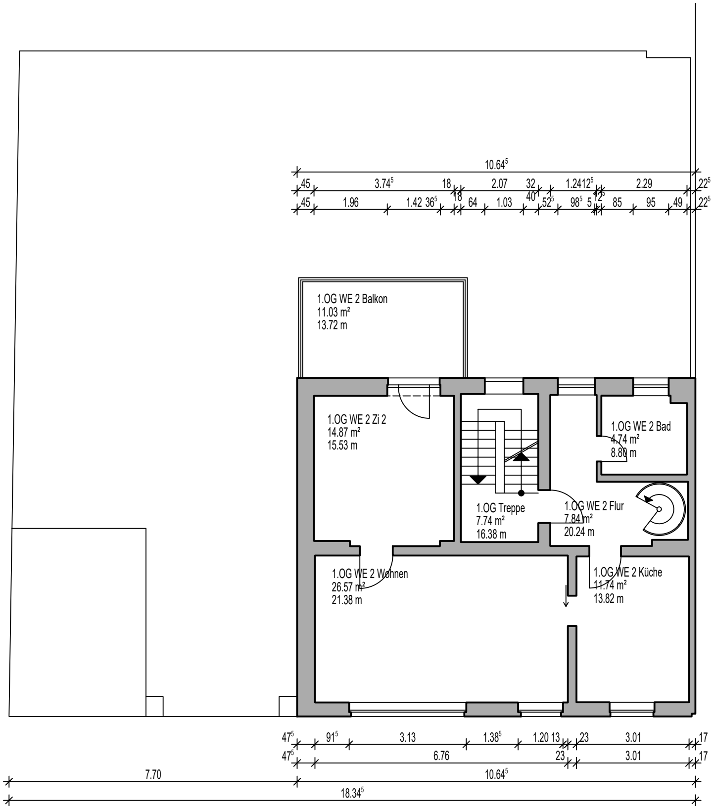
GRUNDRISS 1.OG
