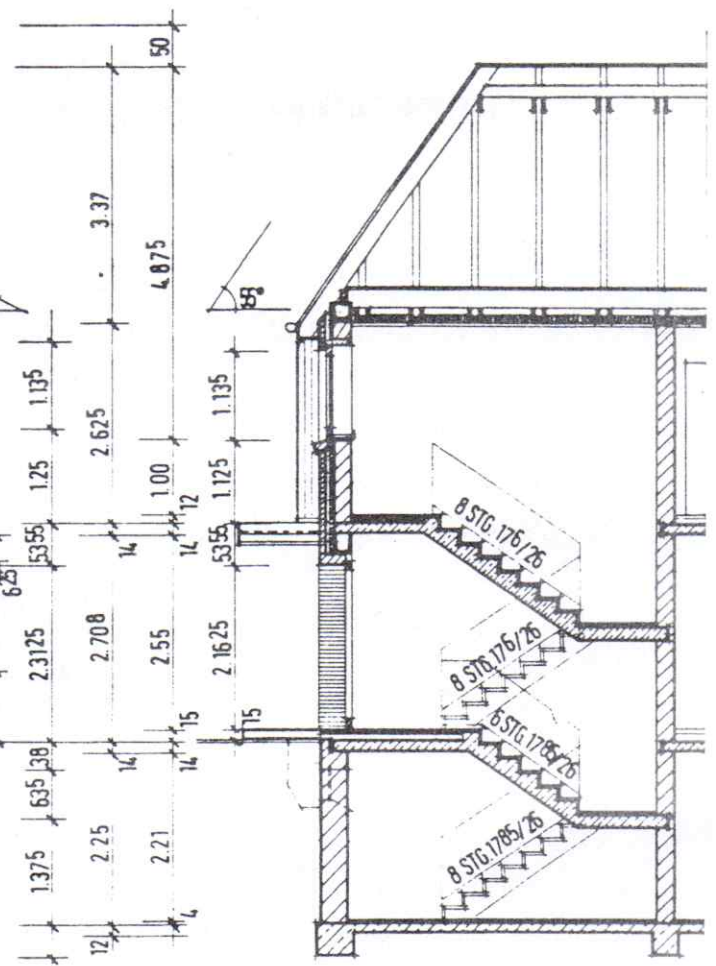
SCHNITT C-D
