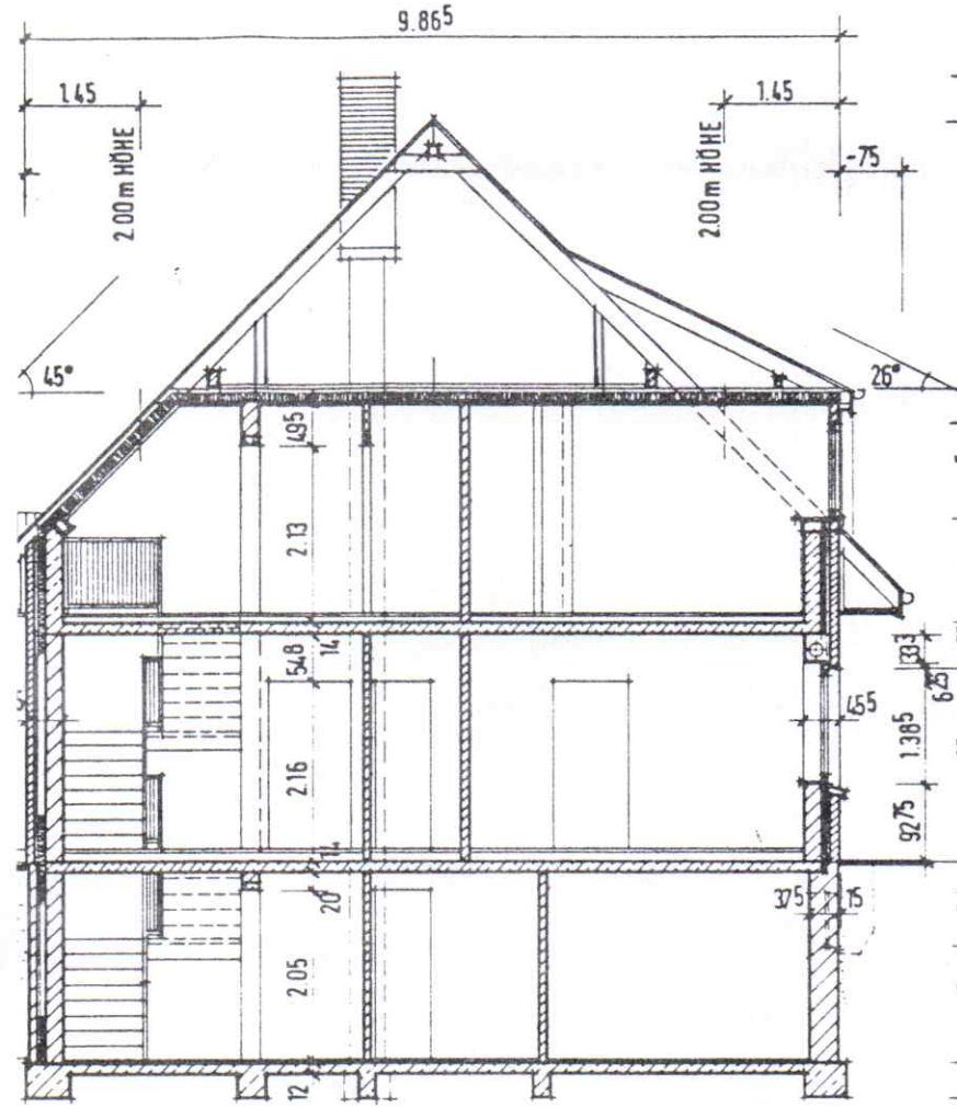
SCHNITT A-B
