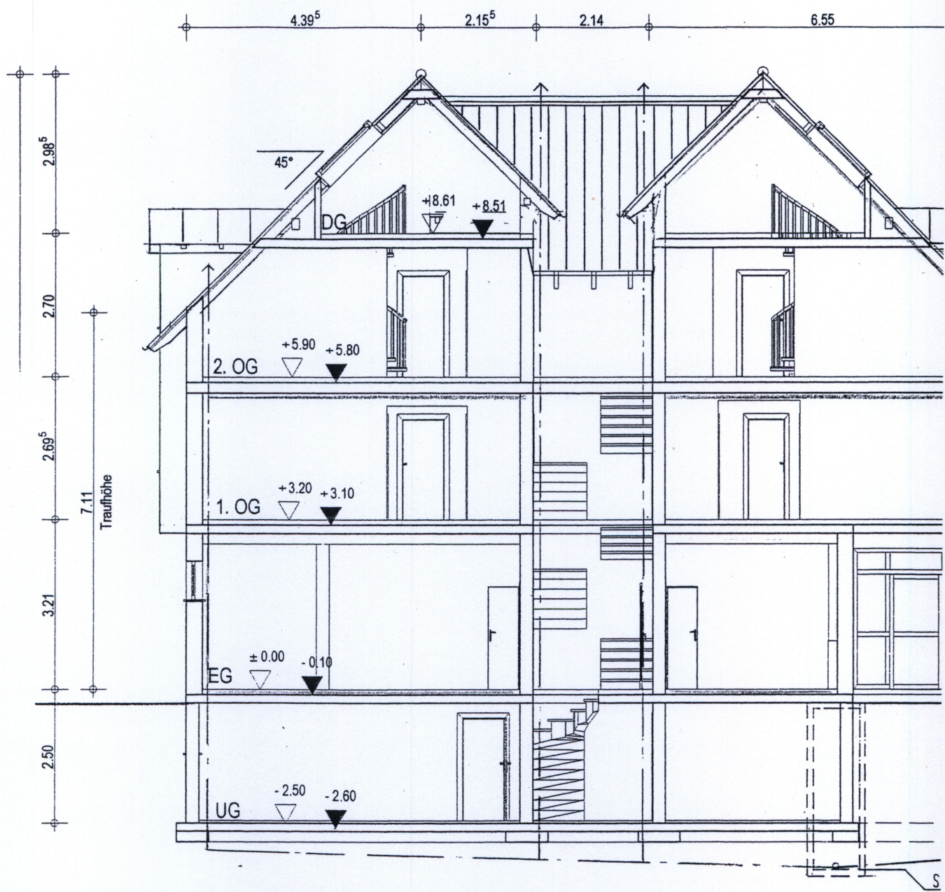
SCHNITT A-A
