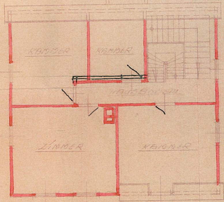
DACH-GESCHOSS
