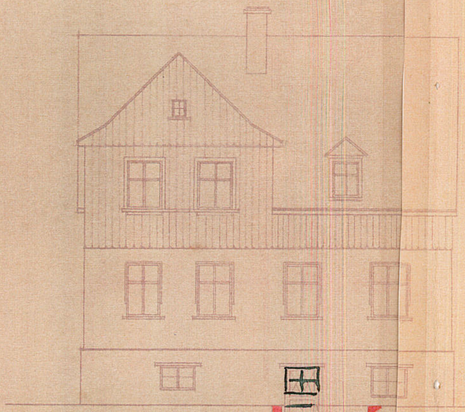
STRASSE-ANSICHT
