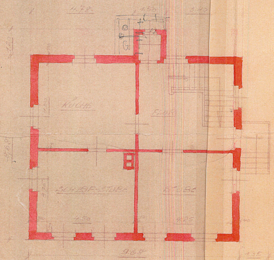
ERD-GESCHOSS
