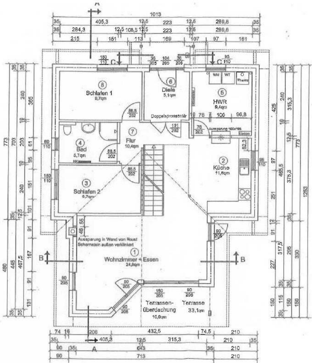
ERDGESCHOSS
