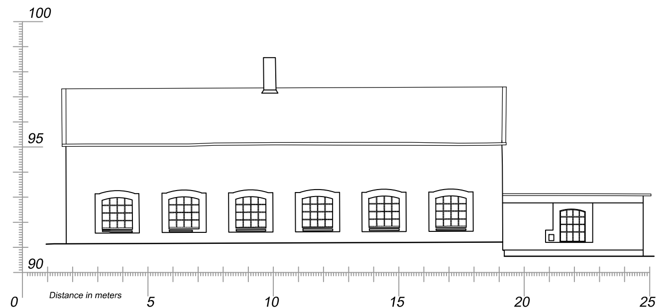
Ansicht 2
