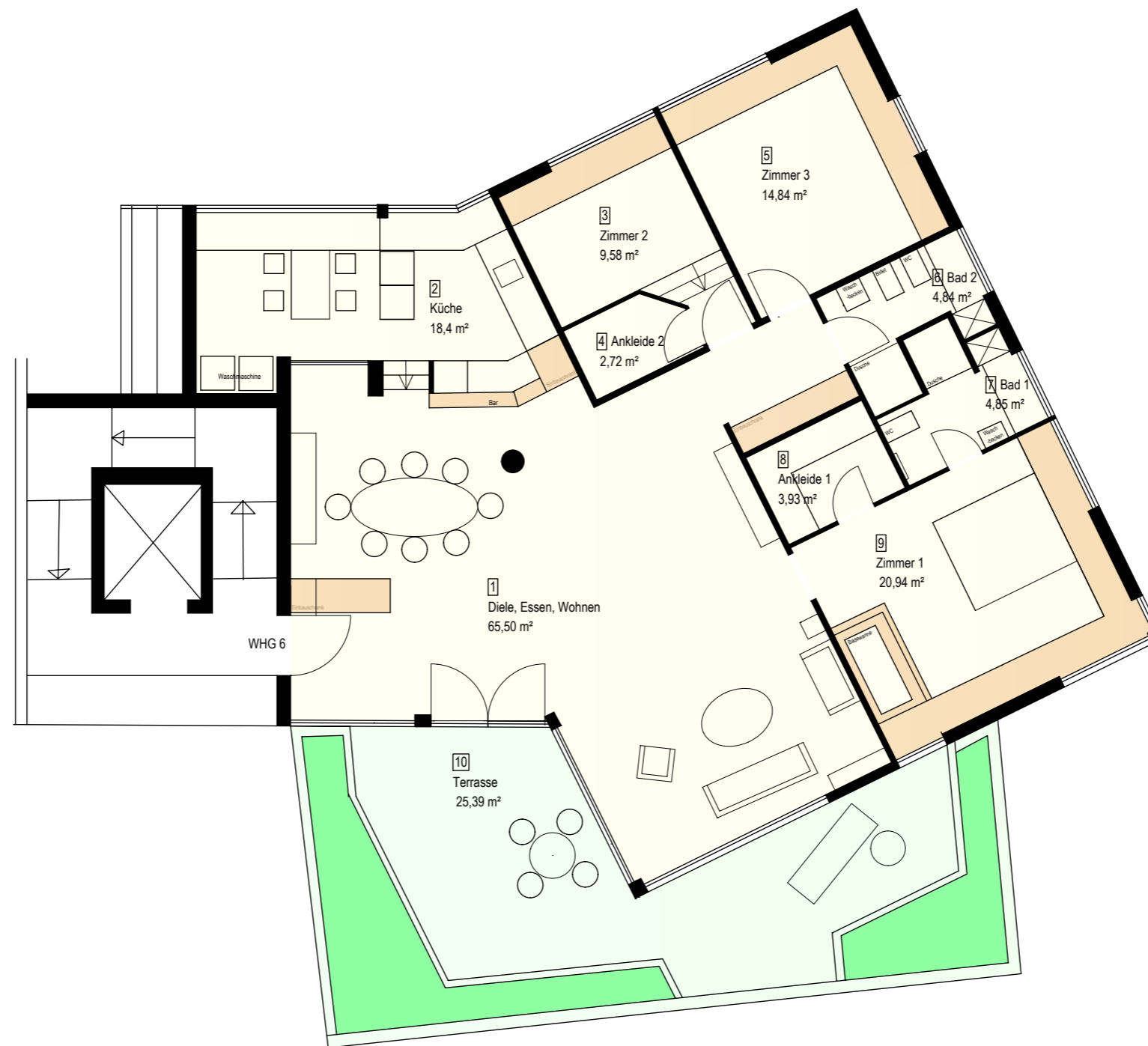
Grundriss: 1.OG WHG 6
