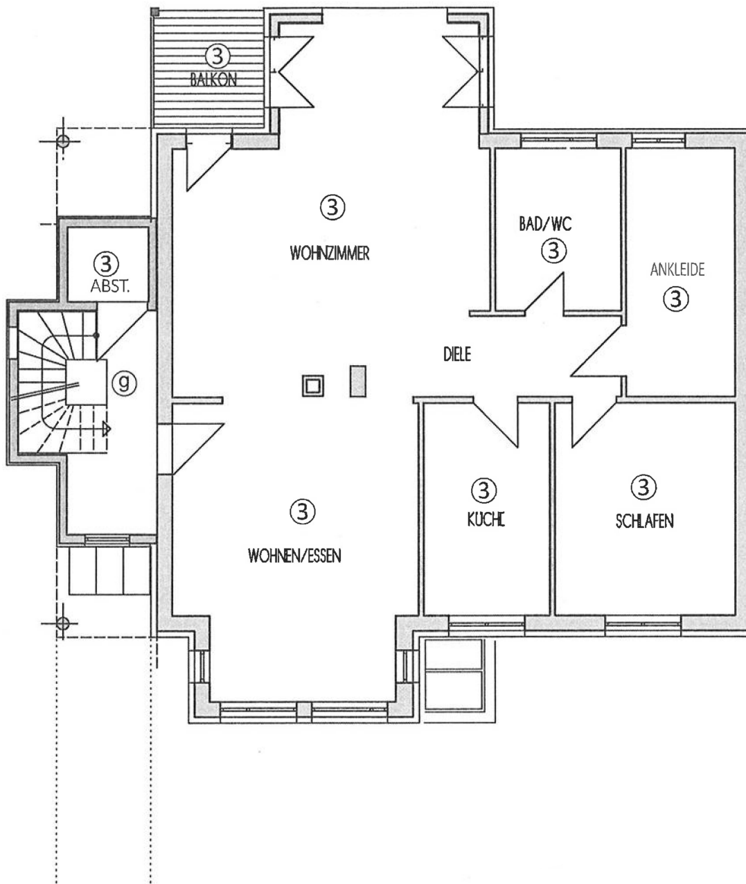
Grundriss 1.OG
