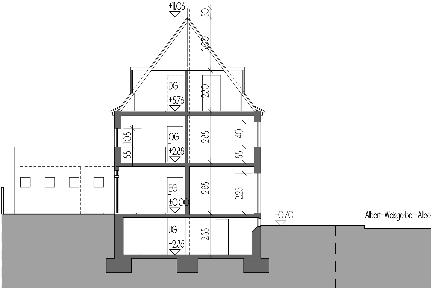
SCHNITT
