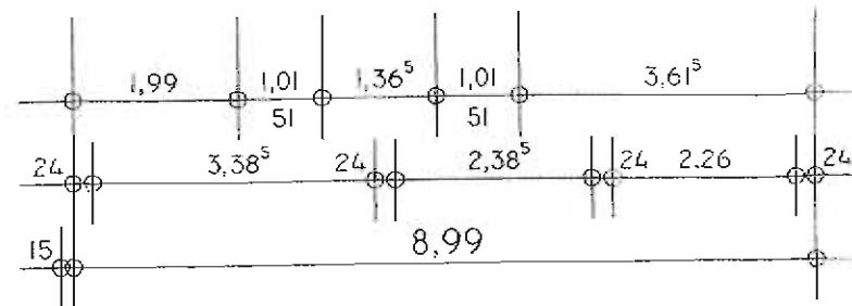
KELLERGESCHOSS M = 1 : 100
