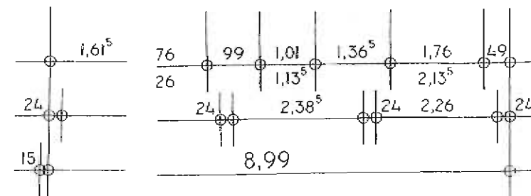
OBERGESCHOSS M = 1 : 100
