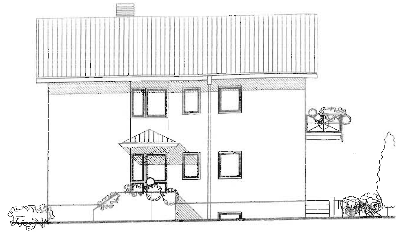
SÜDANSICHT M = 1 : 100
