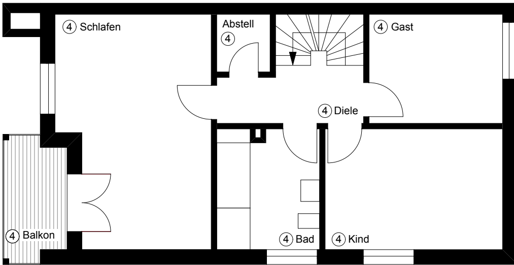
1. OBERGESCHOSS
