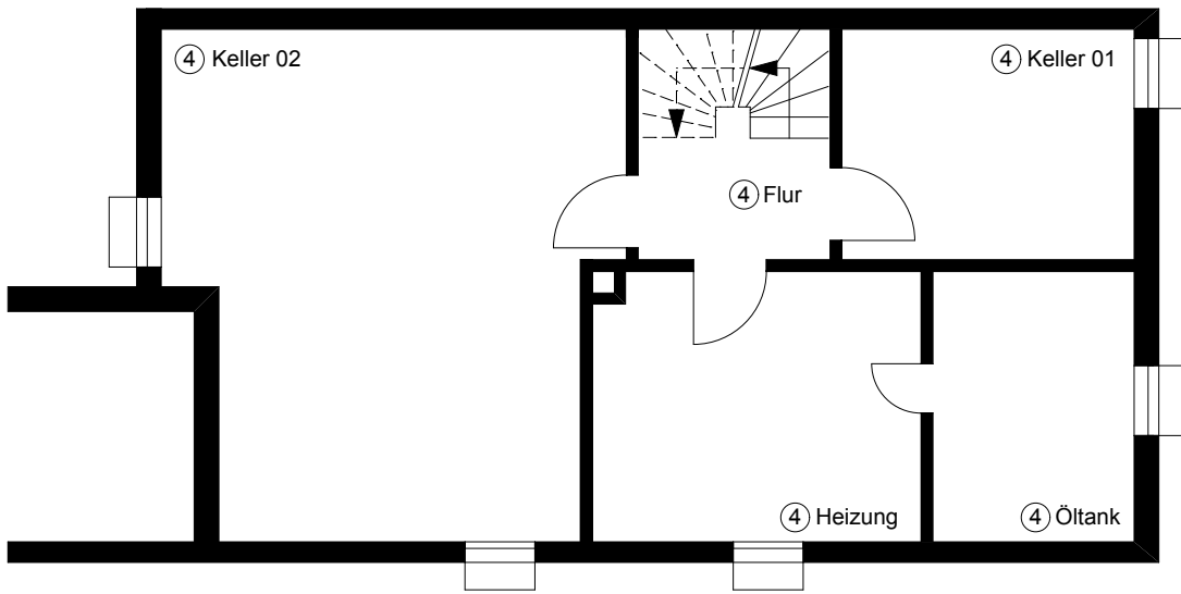
KELLERGESCHOSS
