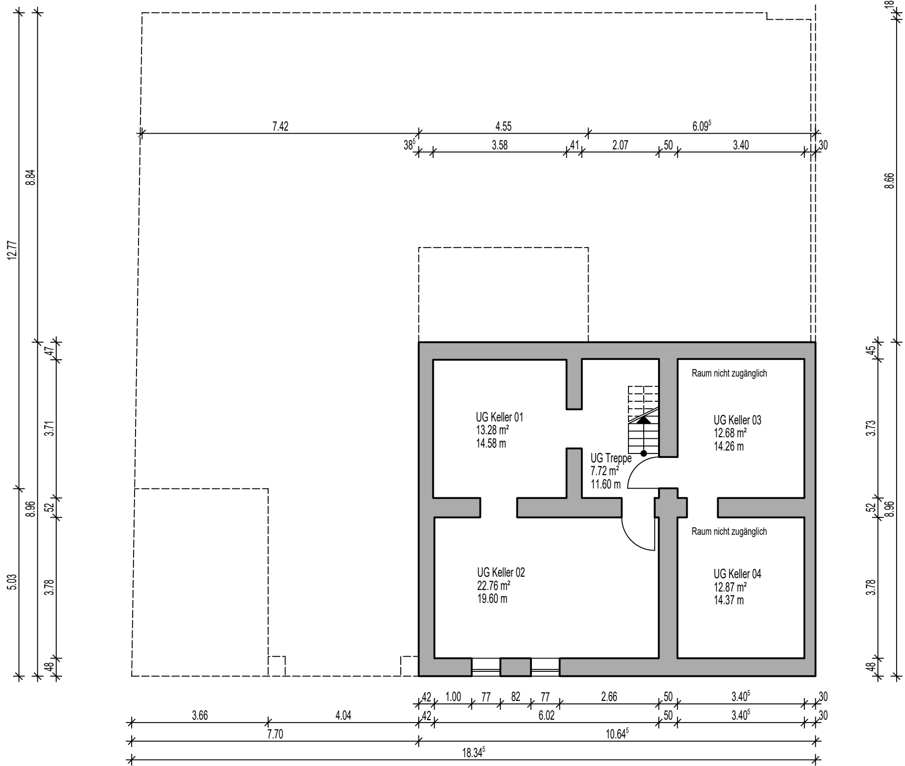
GRUNDRISS UG
