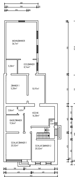
ERDGESCHOSS
