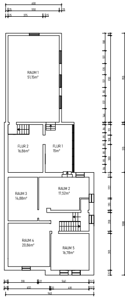
OBERGESCHOSS
