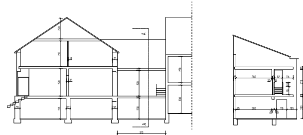
SCHNITT A-A
