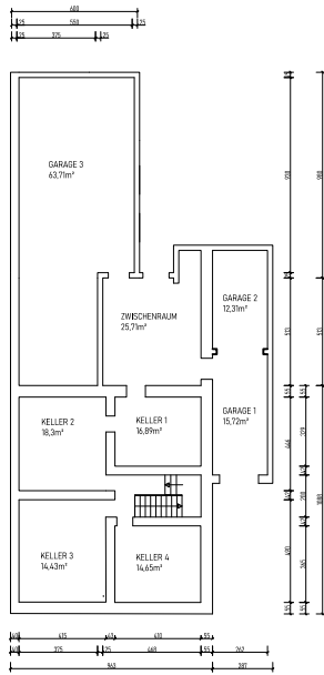
KELLERGESCHOSS
